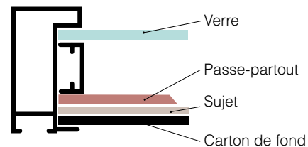
MONTAGE BOÎTE
