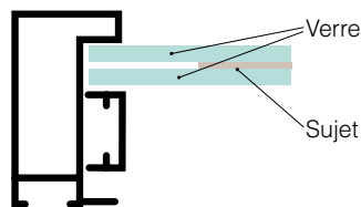
MONTAGE ENTRE-2-VERRES
